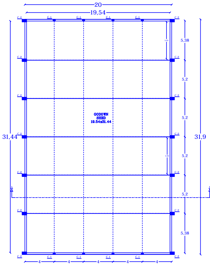
GODOWN PLAN
